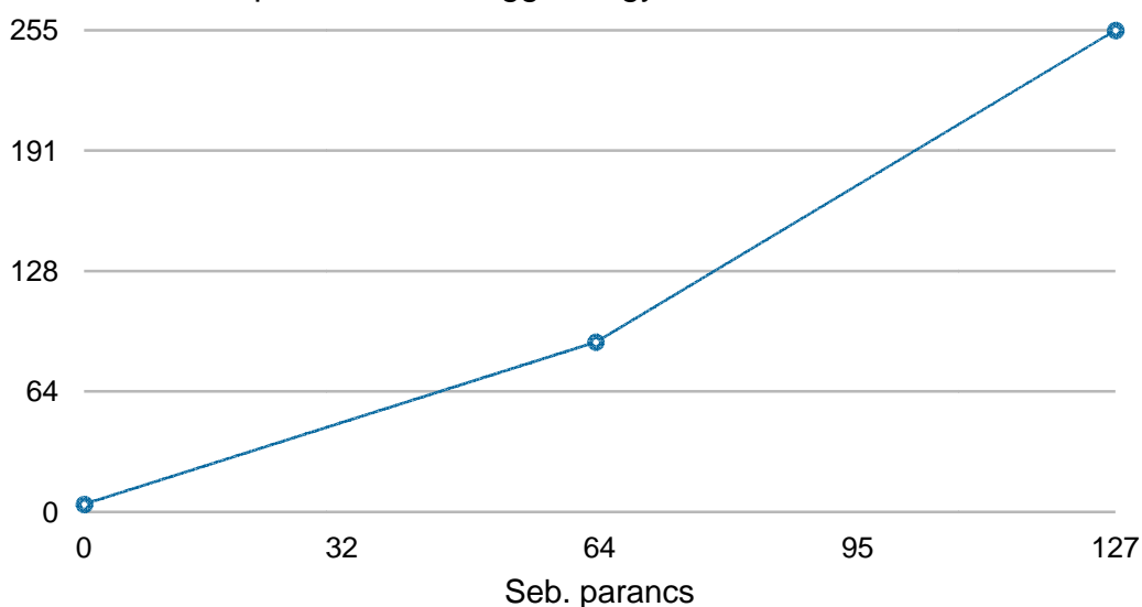
A 3 pontos sebességgörbe gyári beállítása
